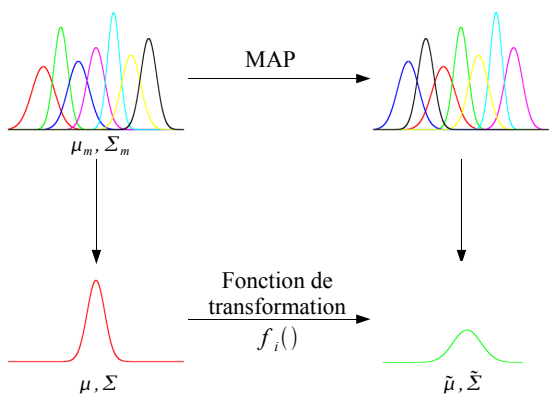
FIG. 2: LIAMAP : principe général de la transformation LIAMAP.
