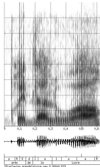
FIG. 2: Spectrogramme de la suite pr'Es de la Loire reconnue comme prøvaloir. On observe une chute presque compløte du mot de, esquisøe uniquement par l'occlusion voisøe du /d/, la phase d'explosion correspond au /l/ de la.
