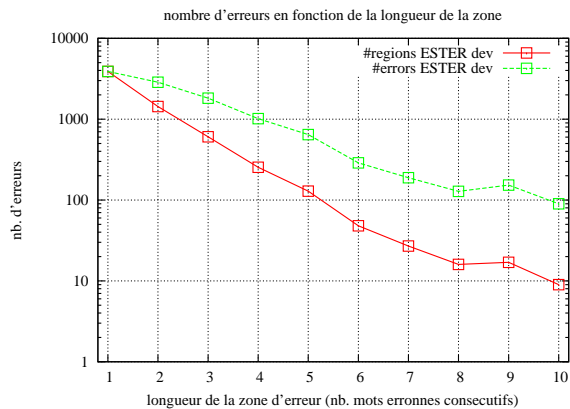
FIG. 1: Nombre d'erreurs et de zones d'erreur en fonction de la longueur de la zone sur le corpus de développement d'ESTER 2004. La longueur d'une zone d'erreur est donnée comme le nombre maximum d'erreurs consécutives (incluant substitution, insertion et omission).
